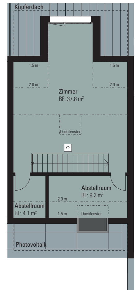
DACHGESCHOSS
