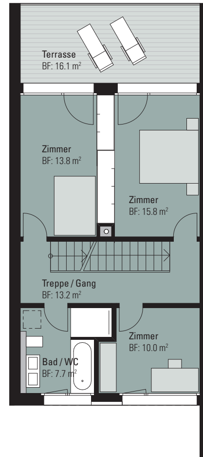
OBERGESCHOSS
